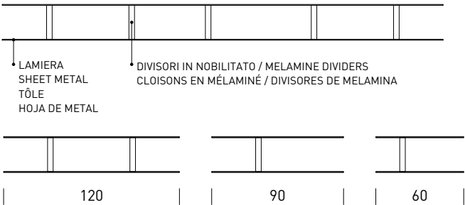
ELEMENTO A GIORNO SOTTOPENSILE / MIDWAY OPEN UNIT ÉLÉMENT OUVERT SOUS LES HAUTS / ELEMENTO ABIERTO BAJO MUEBLE ALTO
